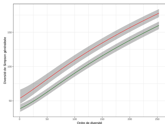
(a) Diversité généralisée de Simpson (nombres effectif d'espèces). Les profils sont distincts, ce qui permet de conclure que la parcelle 6 est plus diverse que la parcelle 18.
