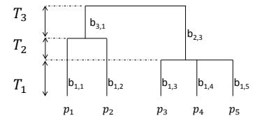
FIGURE 8.1 – Arbre phylogénétique ou fonctionnel hypothétique. Rappel de la figure 7.7(a). 5 espèces sont présentes ( S = 5 ), leurs probabilités notées p_1 à p_5 . Les noms des branches sont affichés.
