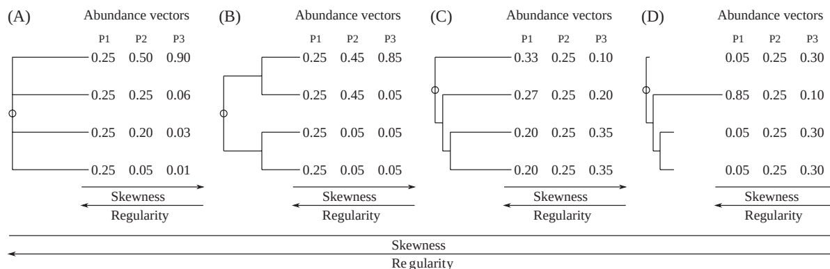
FIGURE 6.2 – Régularité contre irrégularité. Les arbres de A à D sont de plus en plus irréguliers. L'arbre A, parfaitement régulier, est le cadre des mesures classiques de la diversité. La phylogénie étant donnée, trois vecteurs d'abondance (P1 à P3) sont de moins en moins réguliers : dans les cas C et D, la régularité maximale n'est pas obtenue pour des effectifs identiques, mais en augmentant les effectifs des espèces originales (voir Maximum théorique, page 115). La figure est issue de S. Pavoine et M. B. Bonsall (2011). « Measuring biodiversity to explain community assembly : a unified approach ». In : Biological Reviews 86.4, p. 792-812. DOI : 10.1111/j.1469-185X.2010.00171.x, fig. 1.
