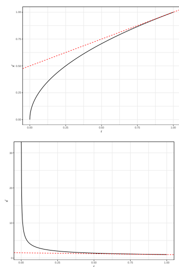
FIGURE 9.2 – Approximation de (\mathbf{Zp})_s^{q-1} par son développement limité au premier ordre pour q = 1.5 en haut ( r = q - 1 ) et q = 0.5 en bas.
