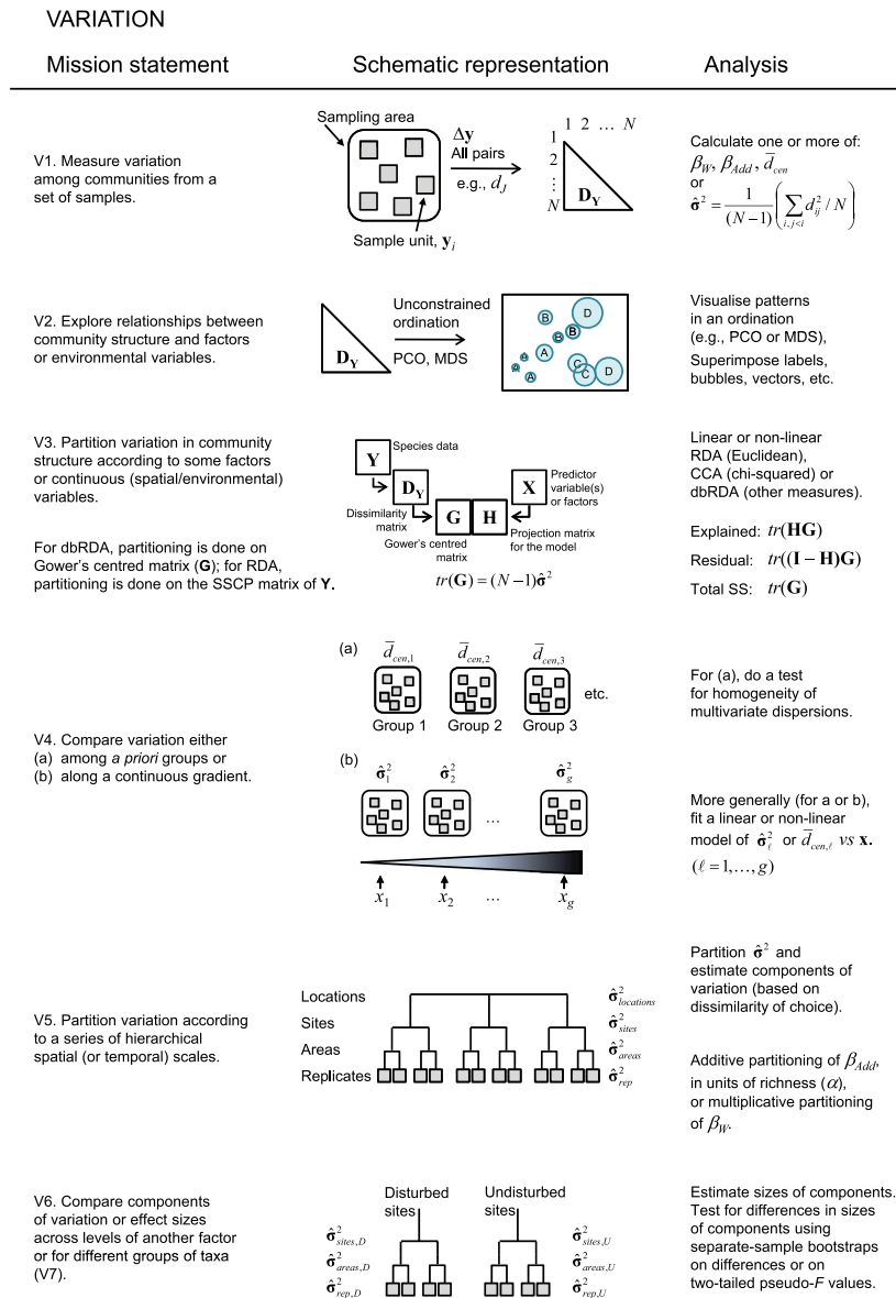
FIGURE 10.2 – Diversité \beta liée à la variation de la composition spécifique. \beta_W est le rapport entre la diversité \gamma et la diversité \alpha , \beta_{Add} leur différence. d_{ij} est la dissimilarité entre les communautés i et j . \hat{\sigma}^2 est la variance de cette dissimilarité, \bar{d} sa moyenne. Si d est une distance euclidienne, \bar{d}_{cen} est la distance moyenne des communautés à leur centre de gravité. (in Anderson et al. a )
