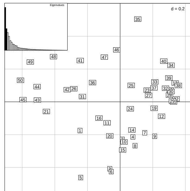
FIGURE 11.8 – PCoA appliquée à la distance de corde des 50 carrés de BCI pour visualiser la diversité \beta .
